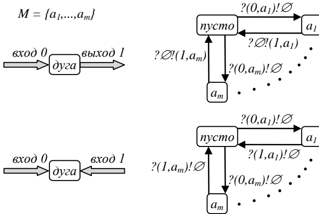
Рис. 5. Автомат очереди длины 1.
