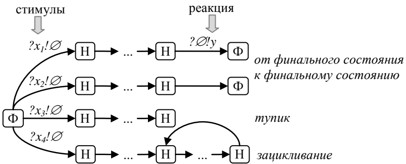
Рис. 3. Типы цепочек переходов в системе после приёма стимула.
