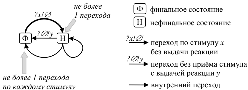
Рис. 2. Типы состояний и переходов автомата системы.
