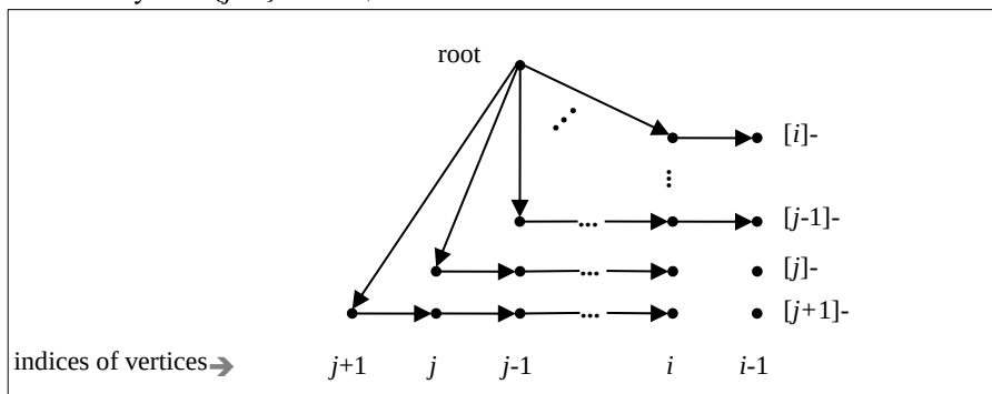
Рис. 5. Склейка сообщений типа 3
